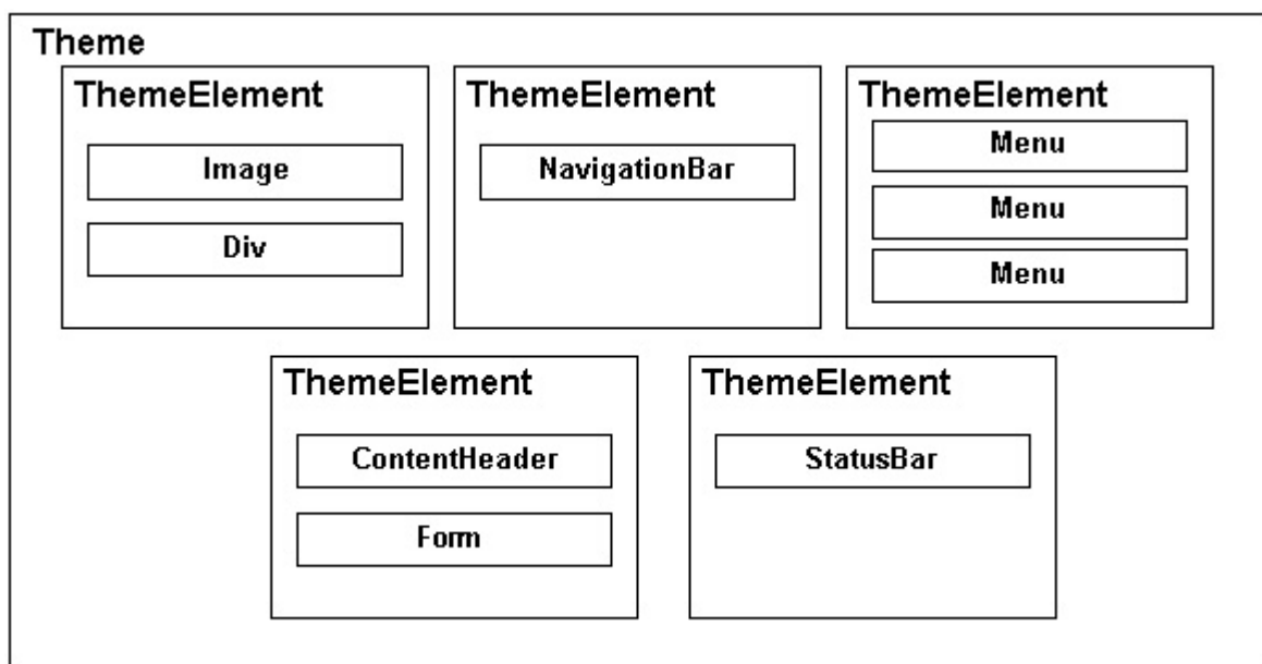
Figura 6 – Estrutura lógica do tema
