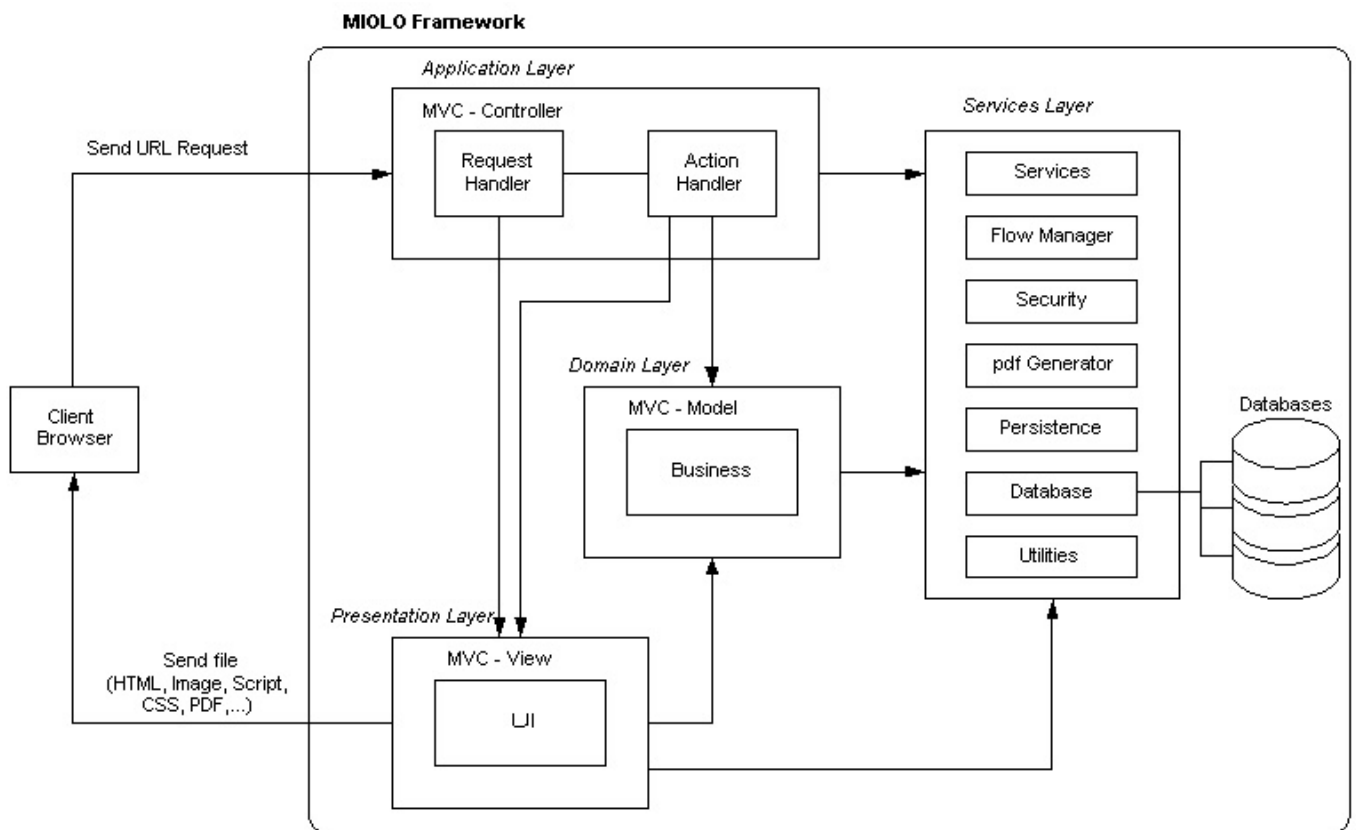
Figura 2 – Padrão MVC
