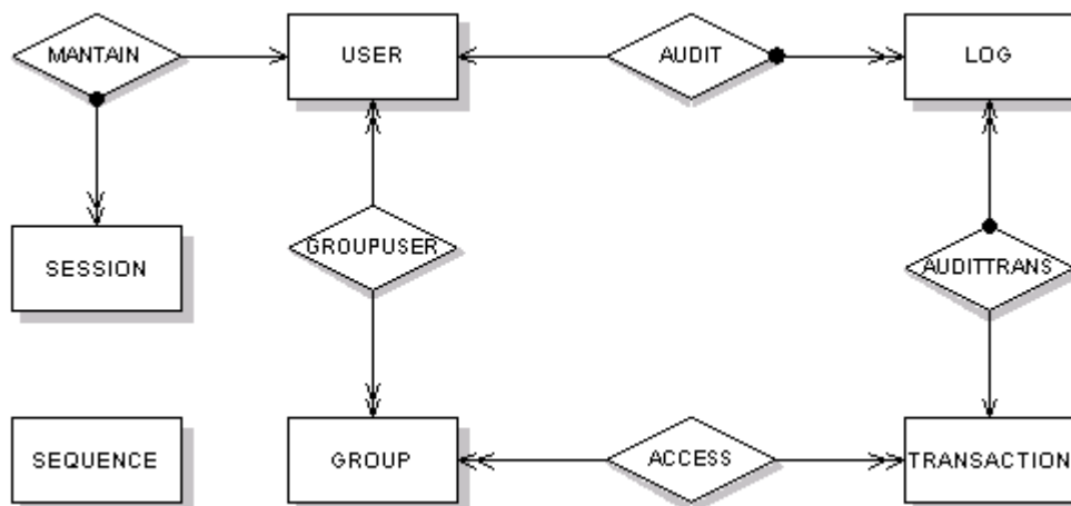
Figura 4 – Base de dados ADMIN
