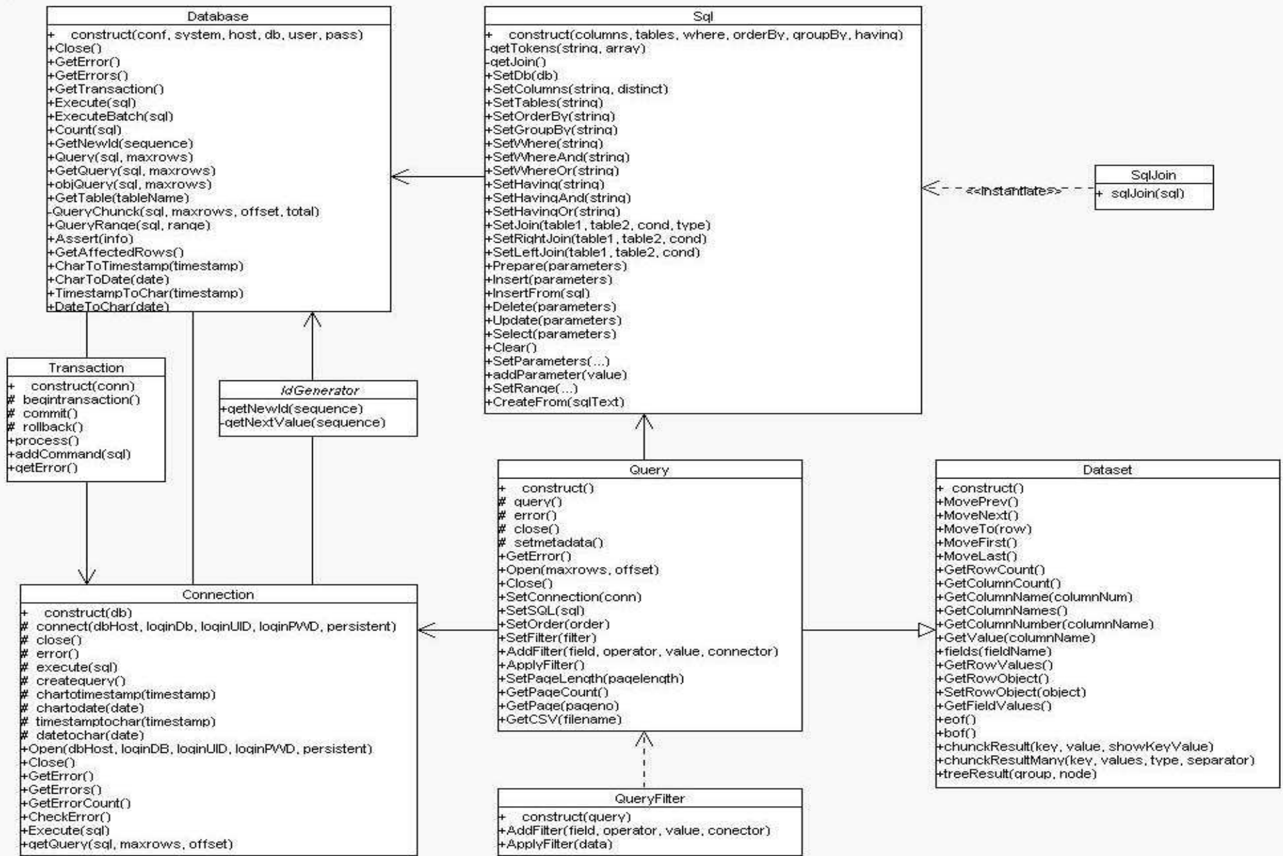
Figura 1 – Visão geral das classes DAO
